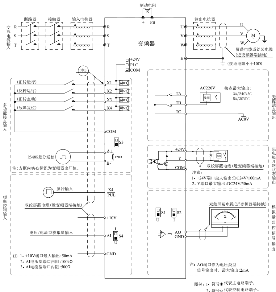
AC10-7.5kW ~ 22kW 功率产品标准接线图
