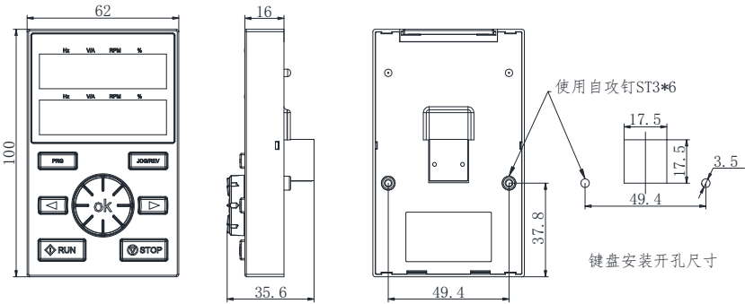
AC10 系列外引双行键盘尺寸
