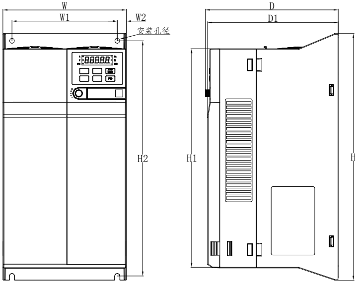
7.5kW-22kW 安装尺寸图
