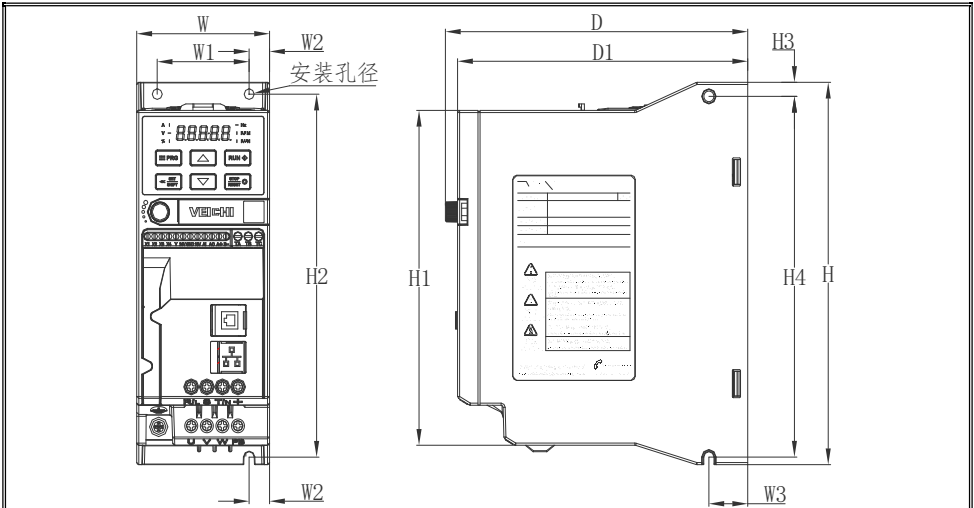
0.4kW-5.5kW 安装尺寸图
