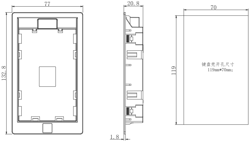
AC10 系列外引双行键盘兜外形及开口尺寸图
